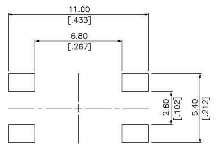
(SCALE 8:1) P.C.B. LAYOUT
