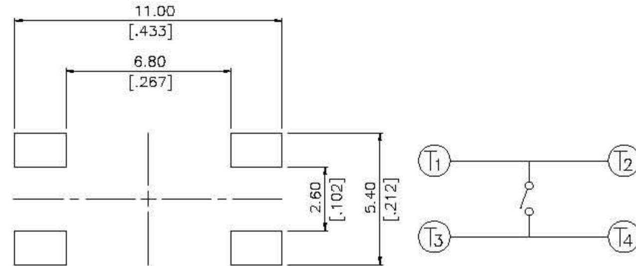
(SCALE 8:1) P.C.B. LAYOUT
