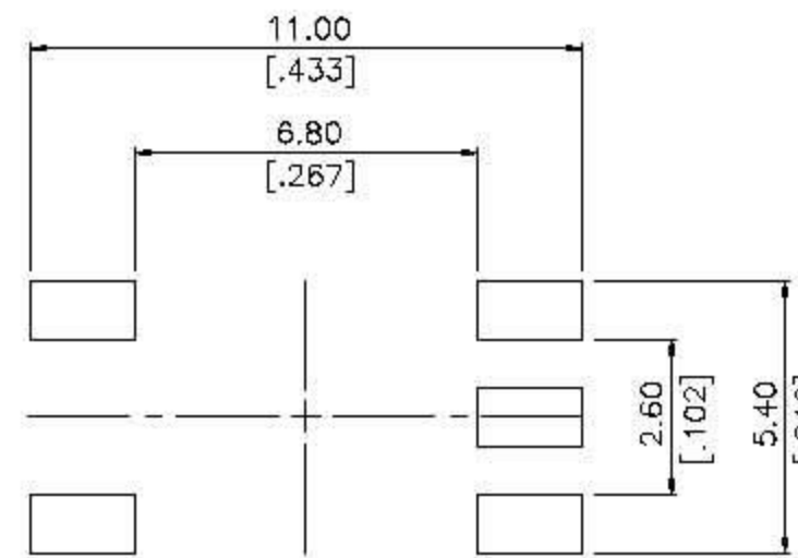
P.C.B. LAYOUT
