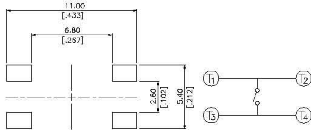
P.C.B. LAYOUT
